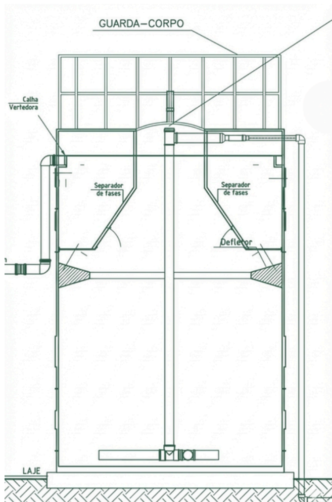
Ilustração 2: vista do equipamento ao nível do terreno.
